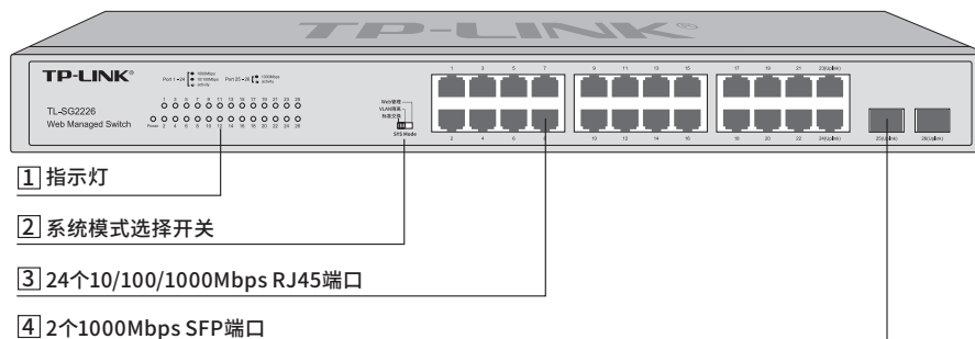
图1-2 TL-SG2226前面板示意图
