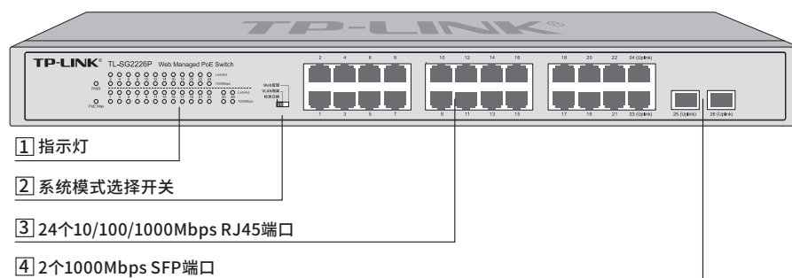
图1-11 TL-SG2226P前面板示意图
