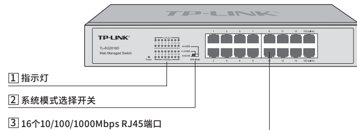
图1-7 TL-SG2016D前面板示意图
