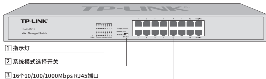
图1-5 TL-SG2016前面板示意图
