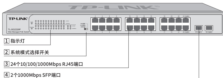
图1-10 TL-SG2226PE前面板示意图
