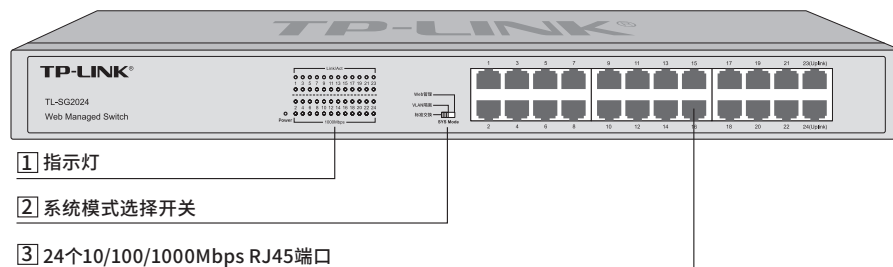
图1-4 TL-SG2024前面板示意图
