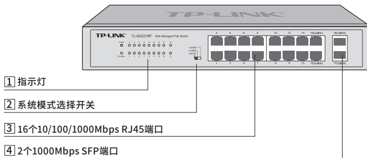
图1-13 TL-SG2218P前面板示意图
