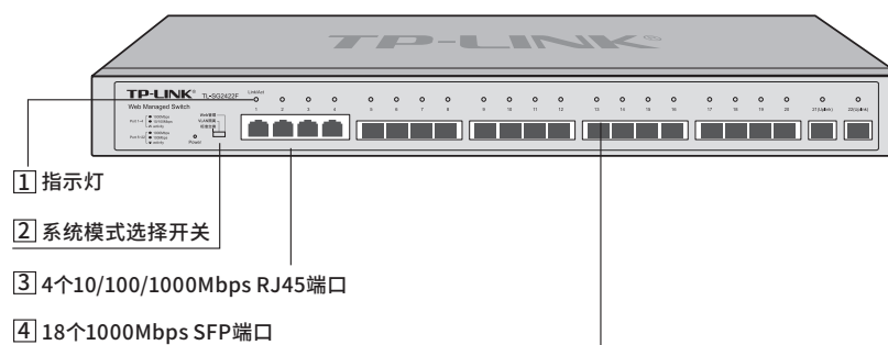
图1-8 TL-SG2422F前面板示意图
