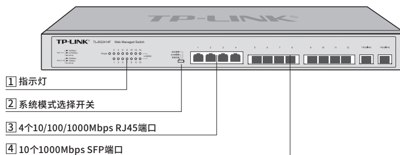
图1-9 TL-SG2414F前面板示意图
