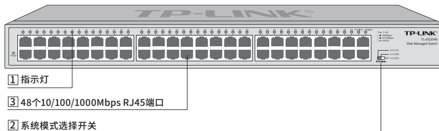
图1-1 TL-SG2048前面板示意图
