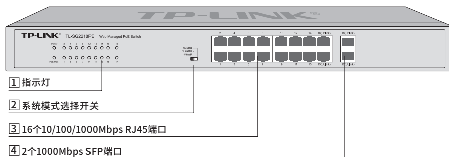
图1-12 TL-SG2218PE前面板示意图
