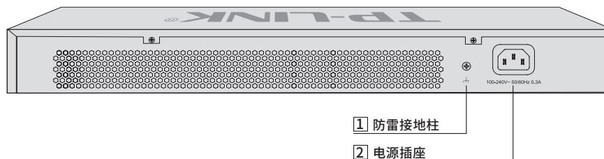
图1-16 后面板示意图
