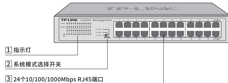
图1-6 TL-SG2024D前面板示意图
