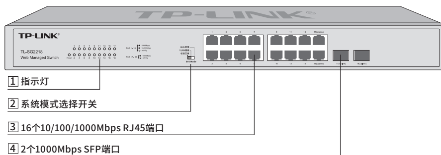
图1-3 TL-SG2218前面板示意图
