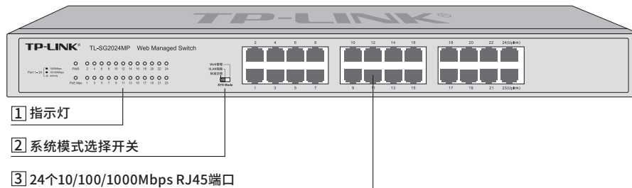
图1-14 TL-SG2024MP前面板示意图
